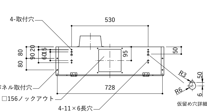
背面取付図
