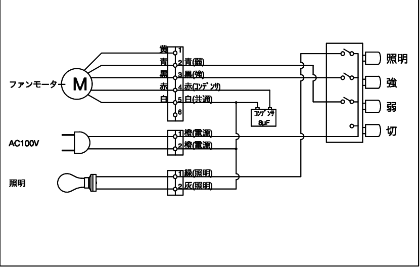
□結線図
