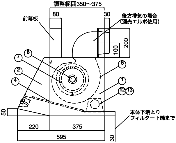
背面取付図
