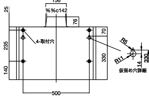
背面取付図
