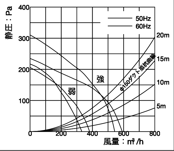
□静圧 - 風量曲線
