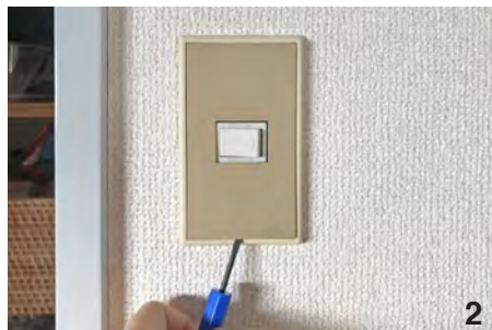
2 外側の枠と表面のプレートの間、下部中央に薄い隙間があるので、そこにマイナスドライバーを差し込み、表面のプレートを手前に持ち上げてはけません。
