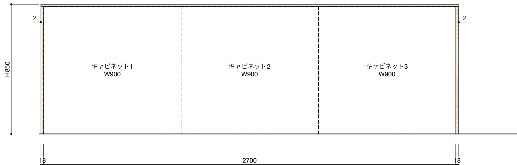
正面図
