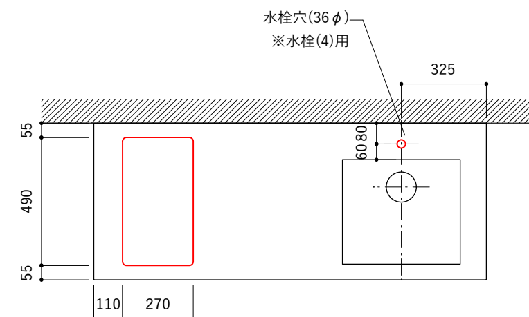
天板開口指示図 開口：Fタイプ
