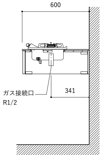
コンロ断面
