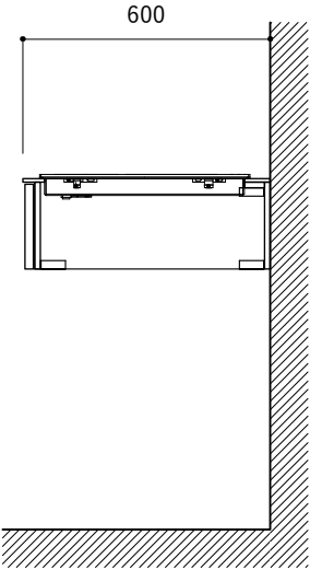
コンロ断面
